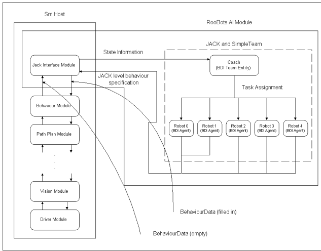
Fig. 1. AI Module
